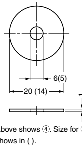
③ Gasket (φ14) ④ Gasket (φ20)
